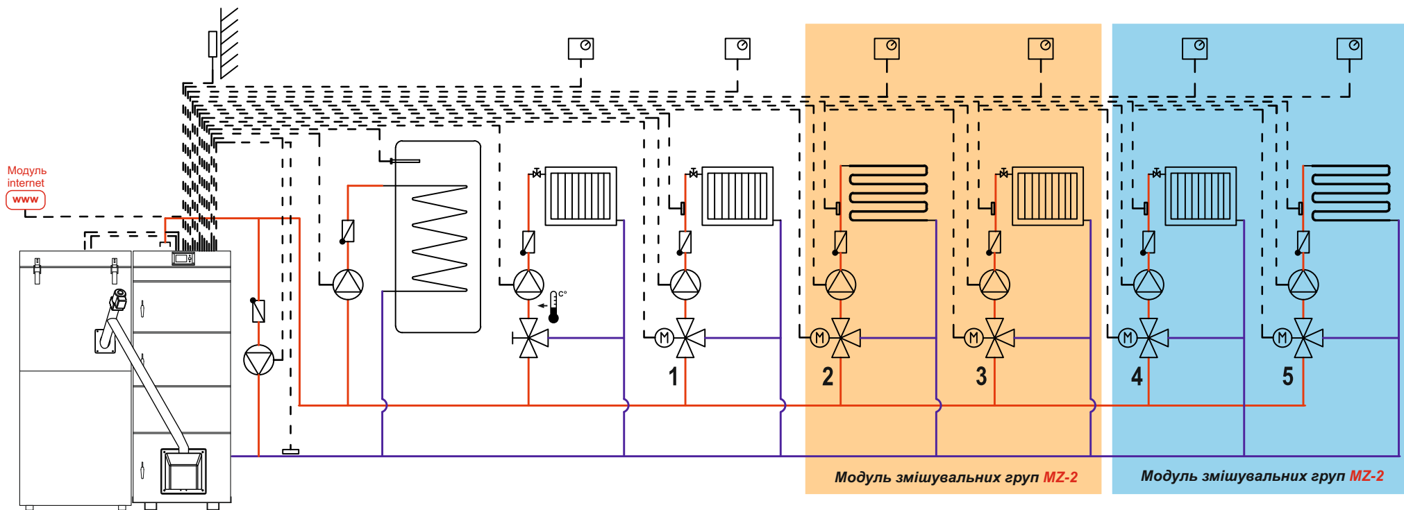
Приклад показує використання автоматики HT-Tronic 900 / HT-Tronic 900 Touch для керування системою опалення та ГВП. Схема не становить проекту інсталяції.
