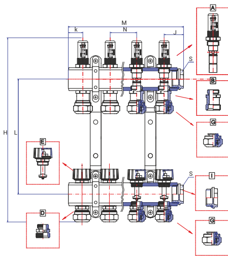
Розподільчий колектор на профілю 1" для підлогового опалення серії 70E / Distributor on 1" profile for underfloor heating of series no. 70E /
