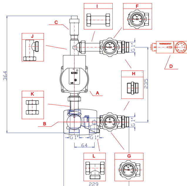
Насосна змішуюча група - серія W40ARA / Circulation mixing unit for distributor - W40ARA series /
