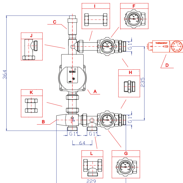
Насосна змішуюча група - серія W40 / Circulation mixing unit for distributor - W40 series /
