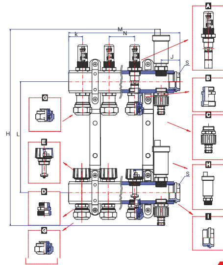
Розподільчий колектор на профілю 1" для підлогового опалення серії 71E / Distributor on 1" profile for underfloor heating of series no. 71E
