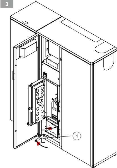
3. Відкривання дверей в камеру попільника. Взяти за ручку (1) підняти її та потягнути на себе.
