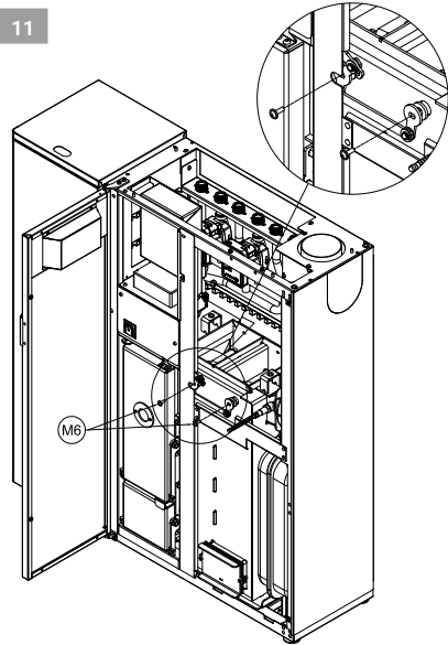
11. Демонтаж механізму приводу турболоізаторів. Відкрутити два гвинти (M6) ключем HEX 5 мм.
