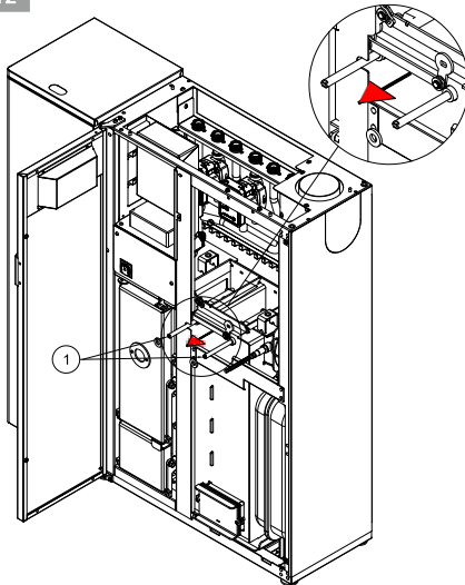
12. Демонтаж турболоізаторів. Витягнути дві направляючі (1) діаметром Ø12 мм.
