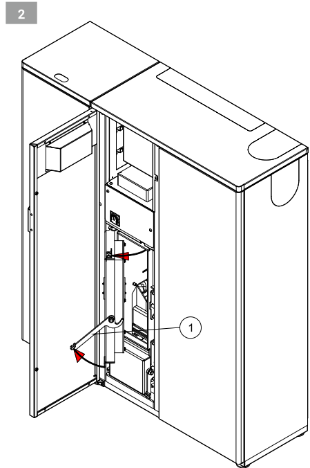
2. Відкривання дверей топки. Взяти за ручку (1) підняти її та потягнути на себе.
