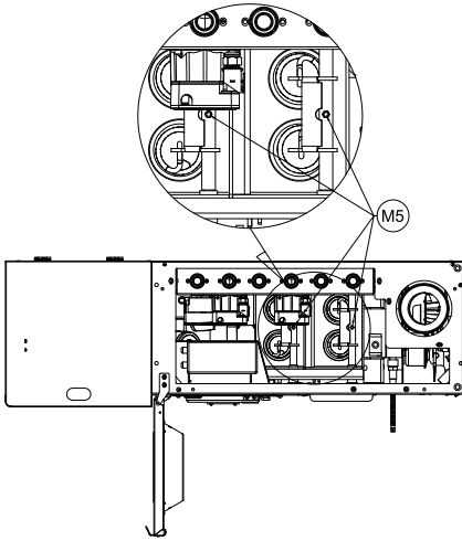
10. Демонтаж турболоізаторів. Відкрутити два гвинти (M5).
