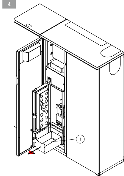
4. Витягування попільника. Взяти ящик (1) і потягнути на себе.
