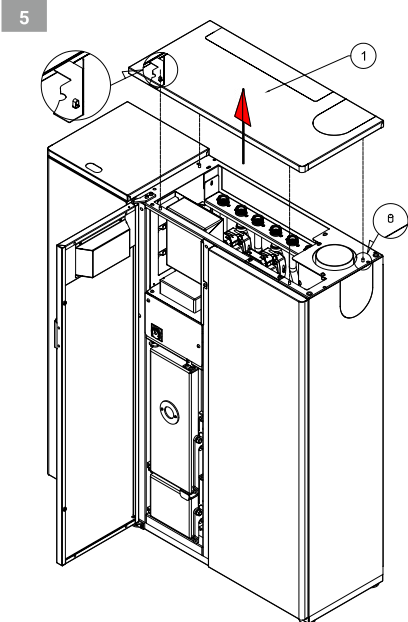
5. Зняття верхньої. Взяти кришку (1) і потягнути вгору
