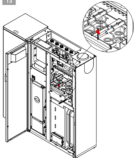
13. Демонтаж турболоізаторів. Витягнути турболоізатори.
