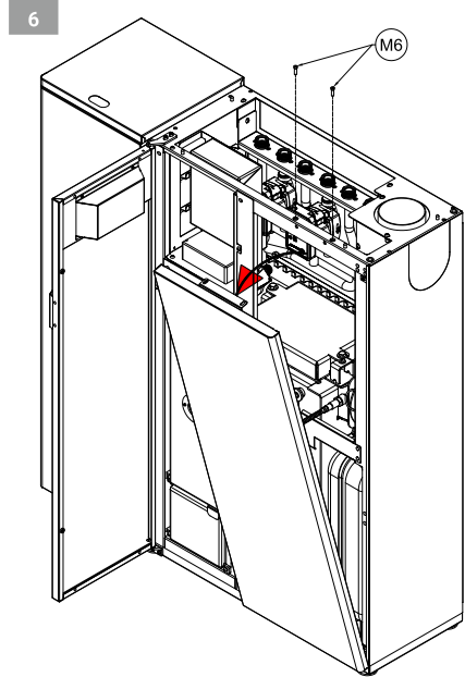
6. Зняття передньої правої кришки. Відкрутити два гвинти (M6) ключем HEX 5 мм і відкрити кришку.
